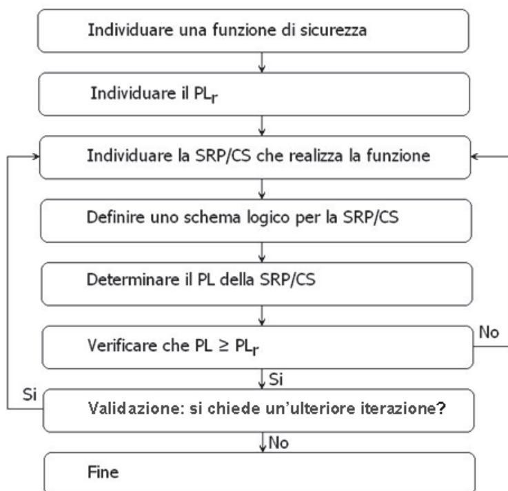
Figura 4: Procedura descritta nella norma ISO EN 13849-1
