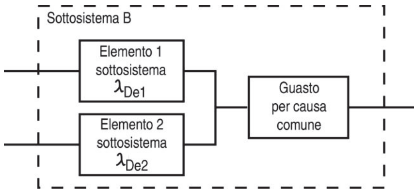
Figura 6: Schema logico Architettura B (EN IEC 62061)
